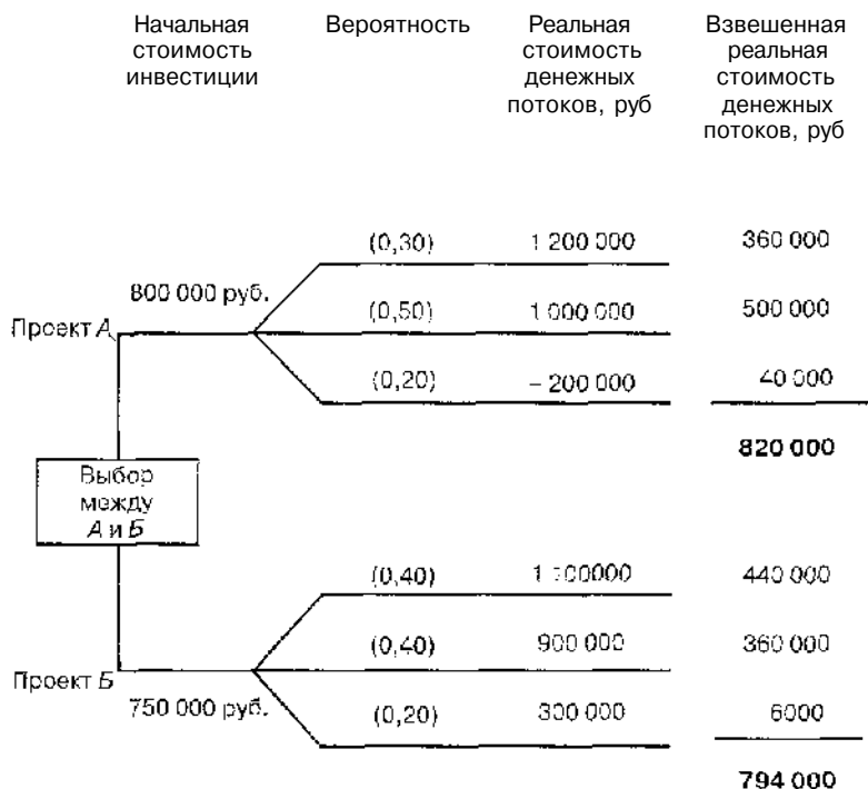
Рис 9.4. Дерево решений
